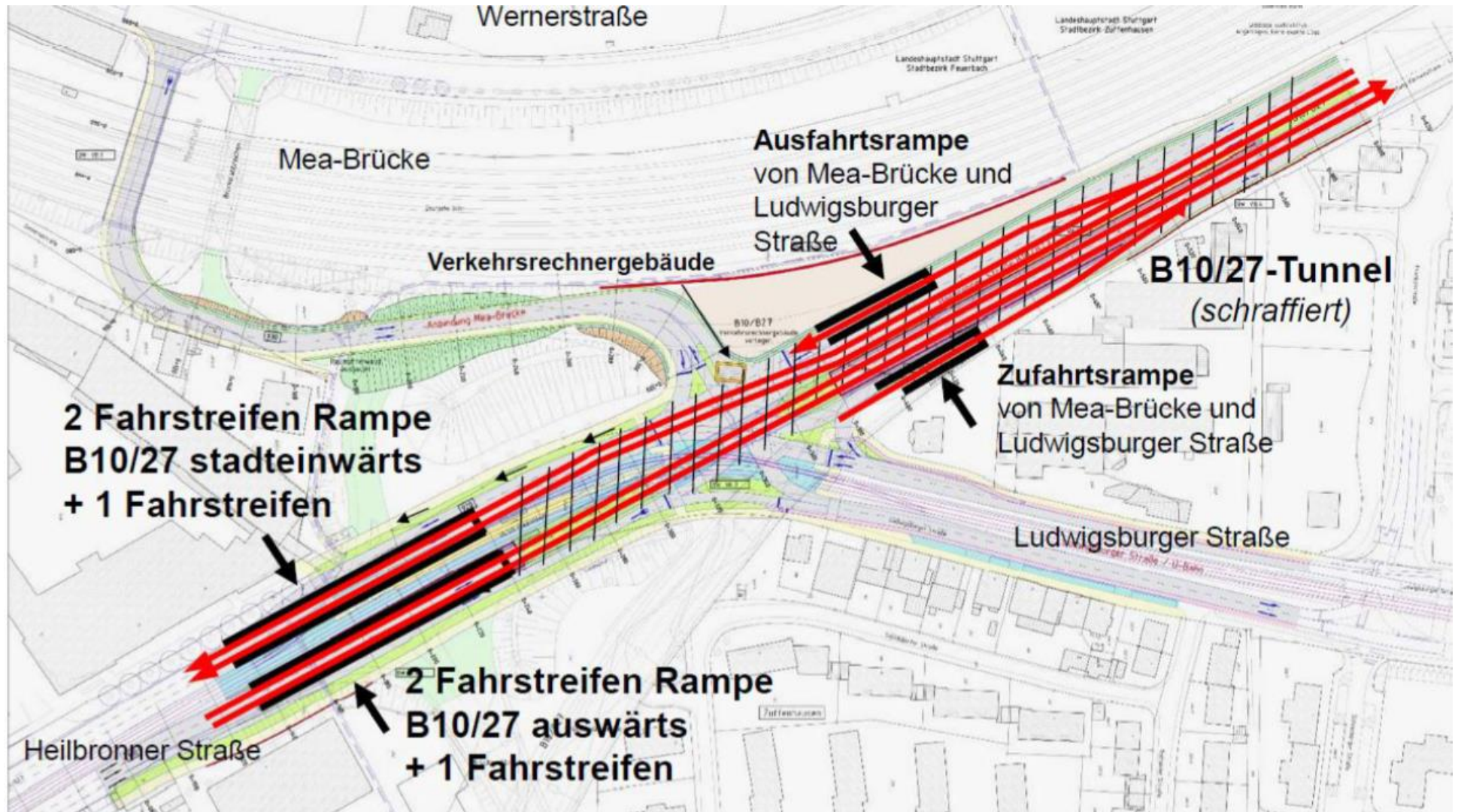
Lageplan Variante 8b.4a, langer Tunnel (600 m) stadtein- und stadtauswärts
