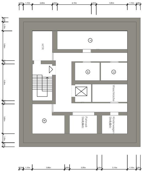
Grundriss UG 2 M 1:100
