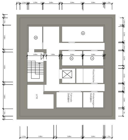
Grundriss UG 1 M 1:100
